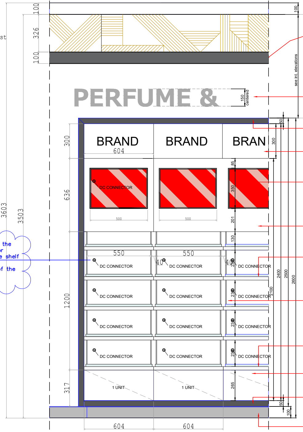
2 ELEVATION scale: 1/20
